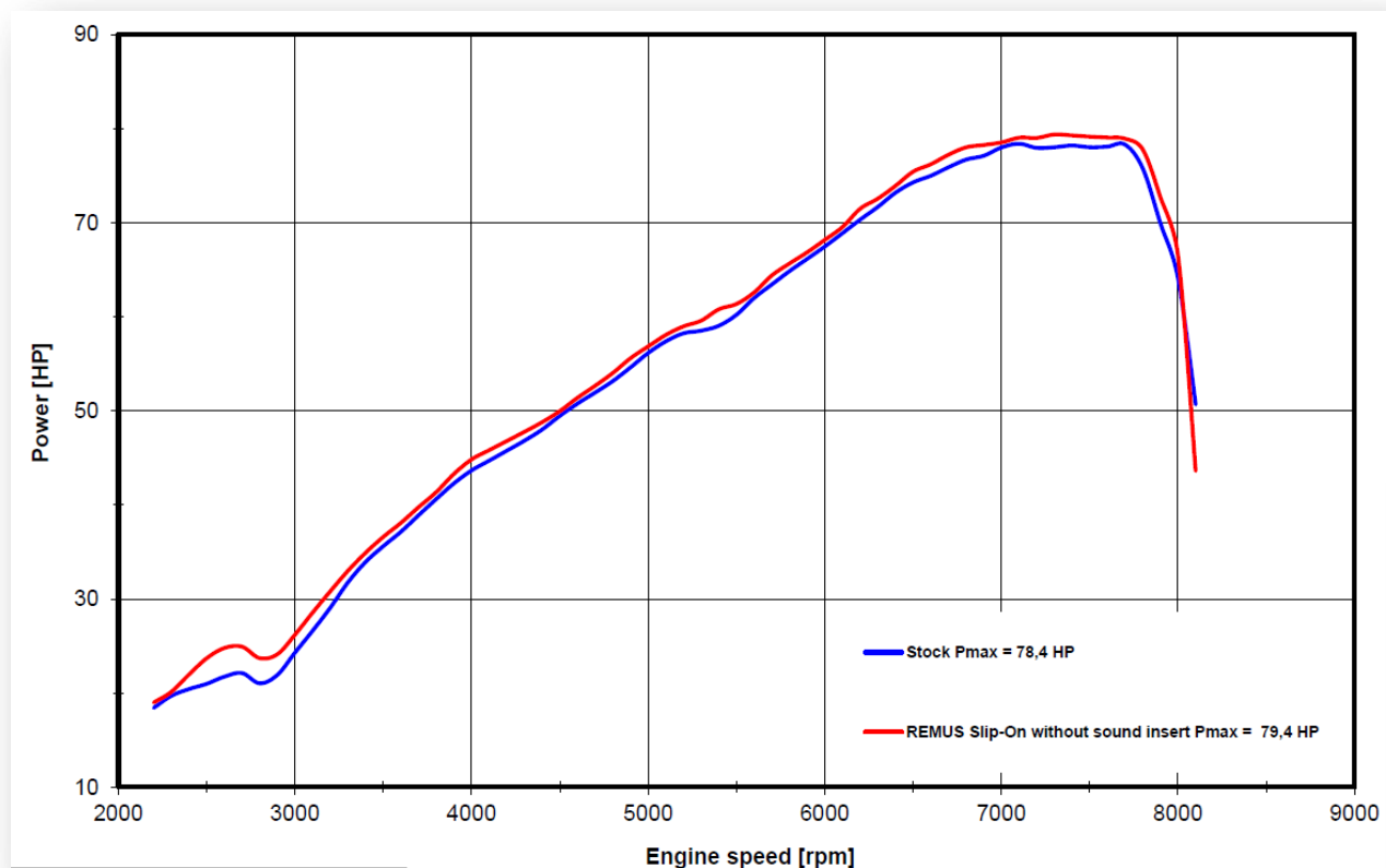
Leistungsdiagramm / Dyno chart – Slip on RACE
