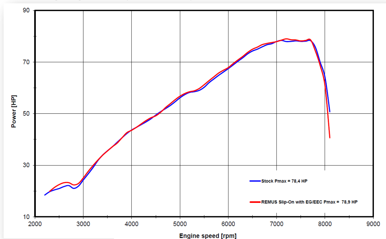
Leistungsdiagramm / Dyno chart – Slip on EG/ABE/EEC
